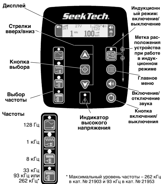
Рис. 4 – кнопочная панель
